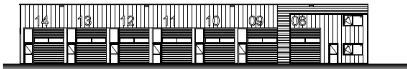
LINKER ZIJGEVEL
