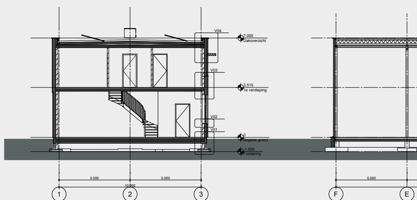
Doorsnede A-A
