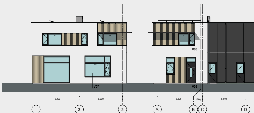
Voorgevel
